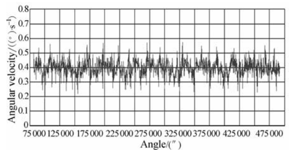
图 9 调频调压驱动下的实测角位置-角速度曲线
