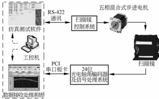
图 7 检测系统组成框图
