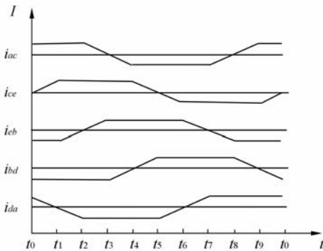
图5 相电流参考波形
