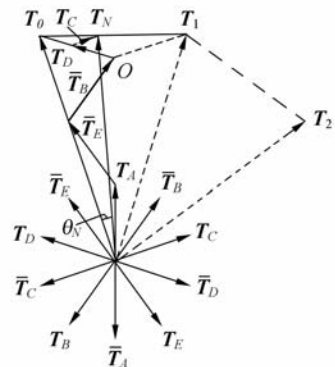
图 4 合成转矩矢量图
