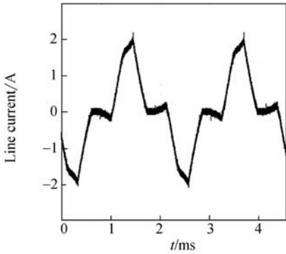
(b) 线电流
