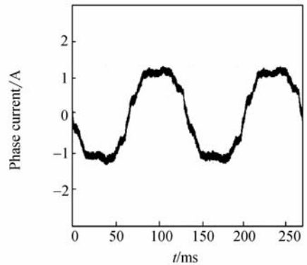
(a) 相电流
