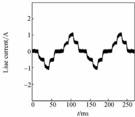
(b) 线电流
