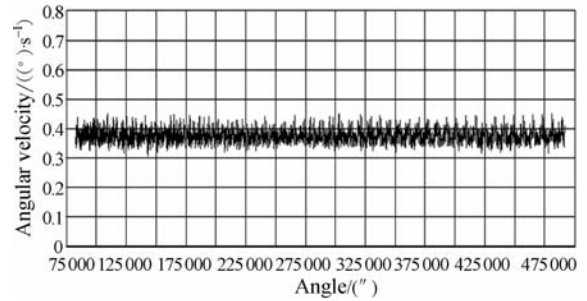
图 8 低速匀速运行实测的角位置-角速度曲线
