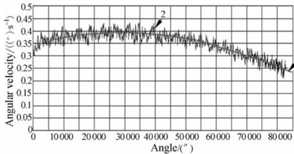
图10 运动补偿模式下实测的角位置-角速度曲线
